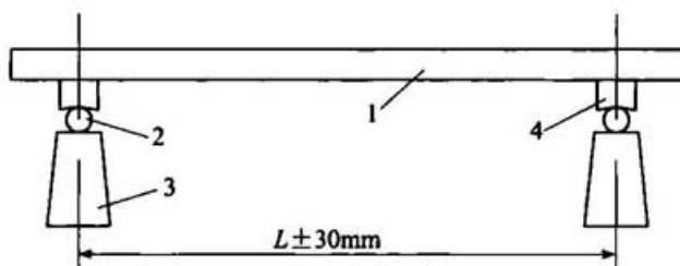
图B. 0. 2 试验用支架示意
