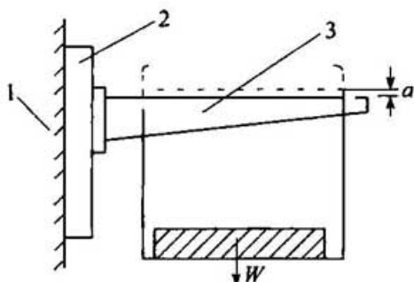
图B. 0. 3-1 支架固定体和定位方式
