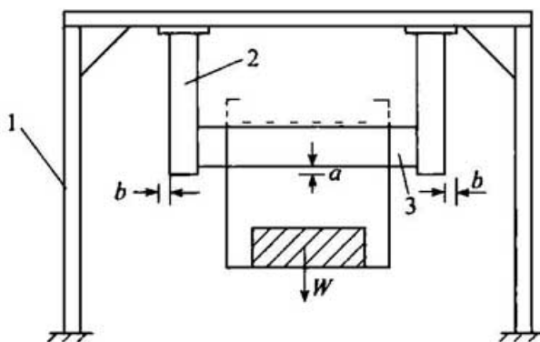
图B. 0. 3-3 吊架固定体和定位方式
