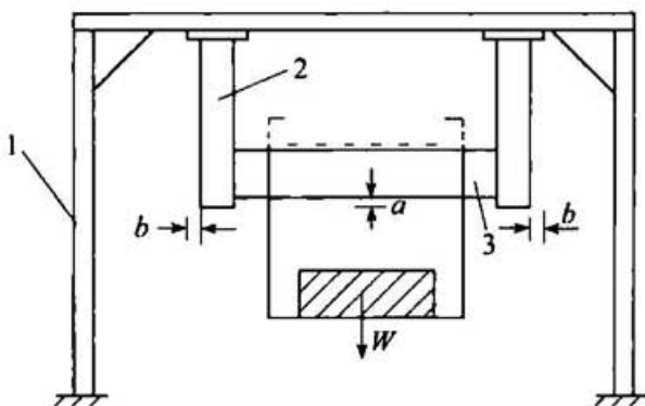
图B. 0. 3-2 支架固定体和定位方式
