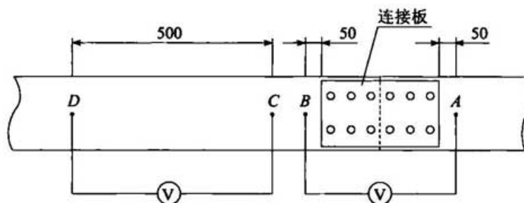
图C. 0. 2 电气连续性试验布置
